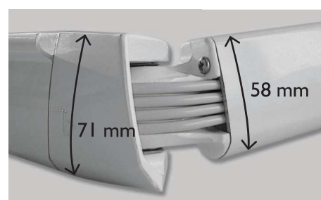
Ramena markýzy B-28 Elite se 4 kabely pro ještě větší vypnutí látky.
