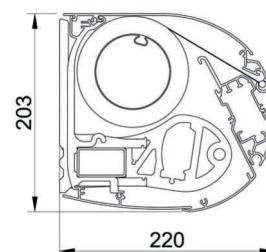
B-35 AUTOMATICKÝ VOLÁN
