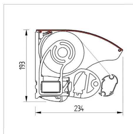
B34 S KRYTÍM
