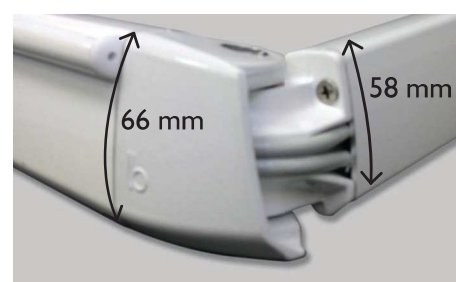
Obdélníková ramena (výška 66mm) s dvojkabelem udržují stále napjatou látku.
