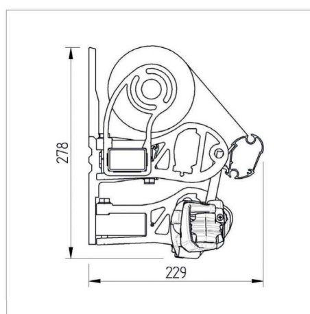
B-34 XL SE SKŘÍŽENÝMI RAMENY
